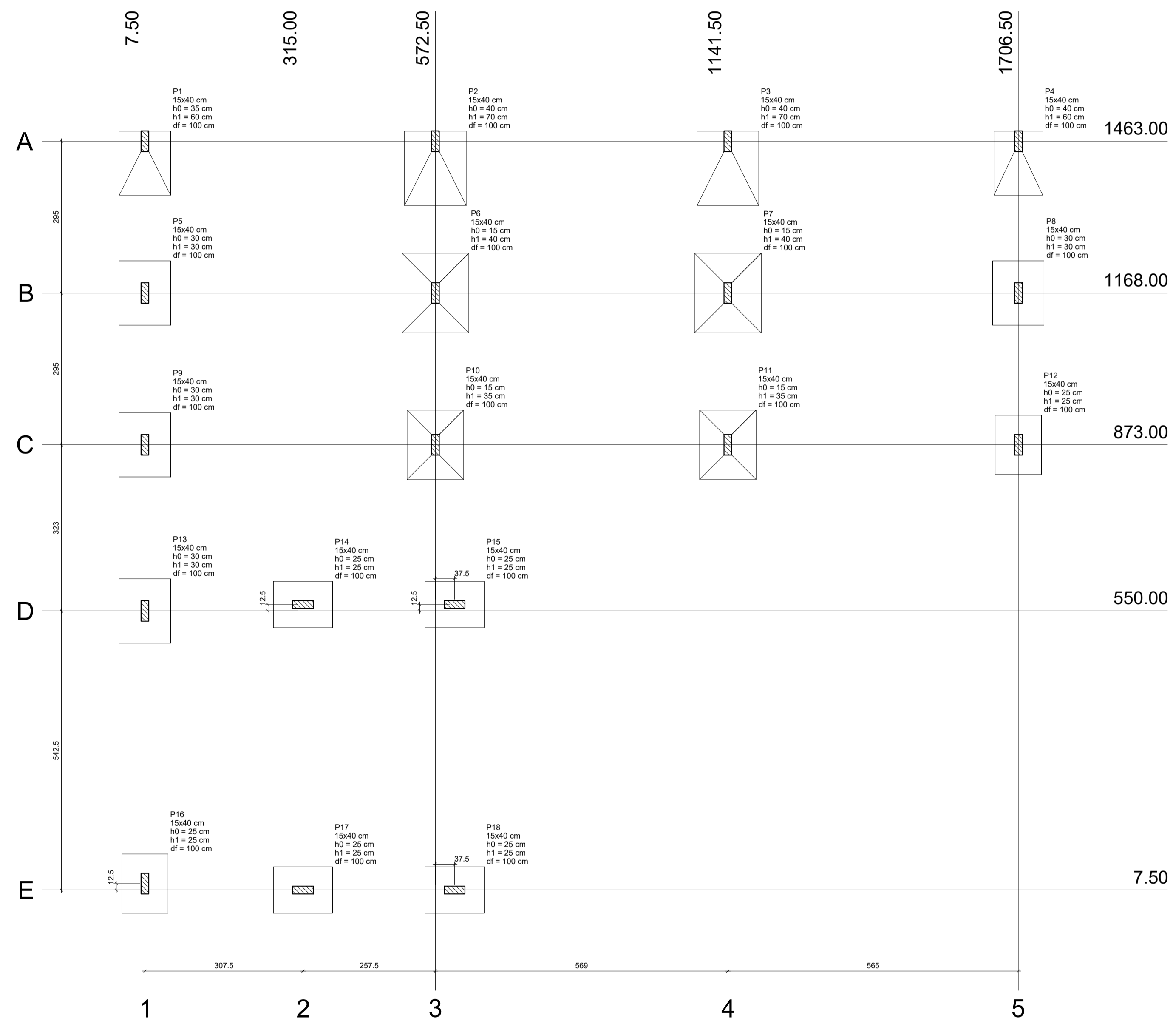
Planta de locação escala 1:50
