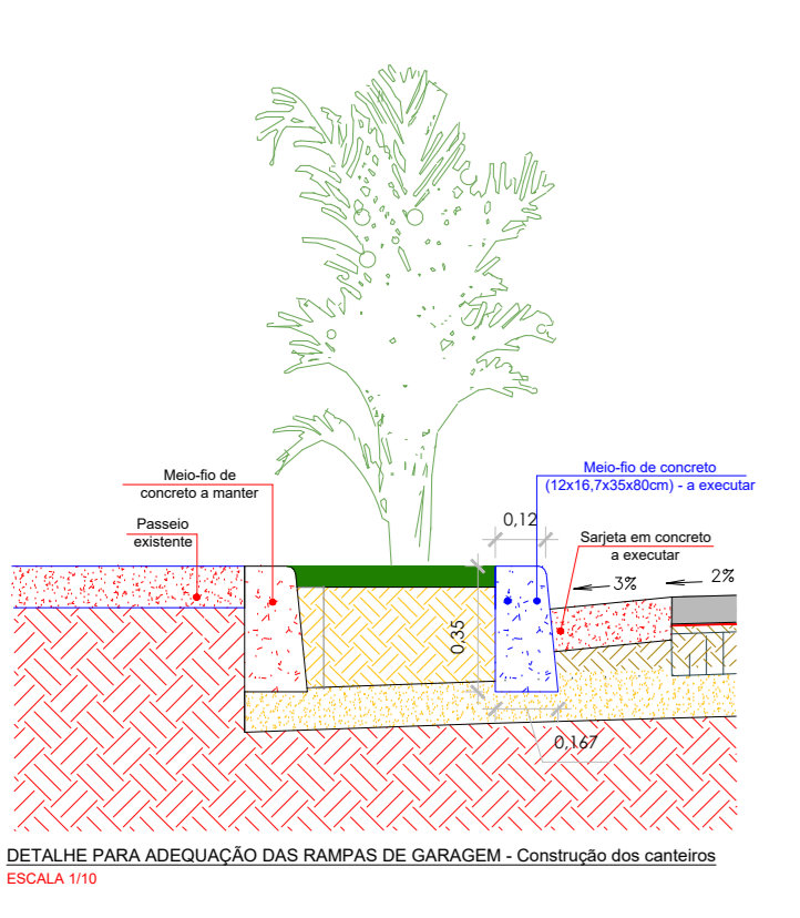
CORTE TRANSVERSAL DO DETALHAMENTO DA RAMPAS DE GARAGEM E CANTEIROS
