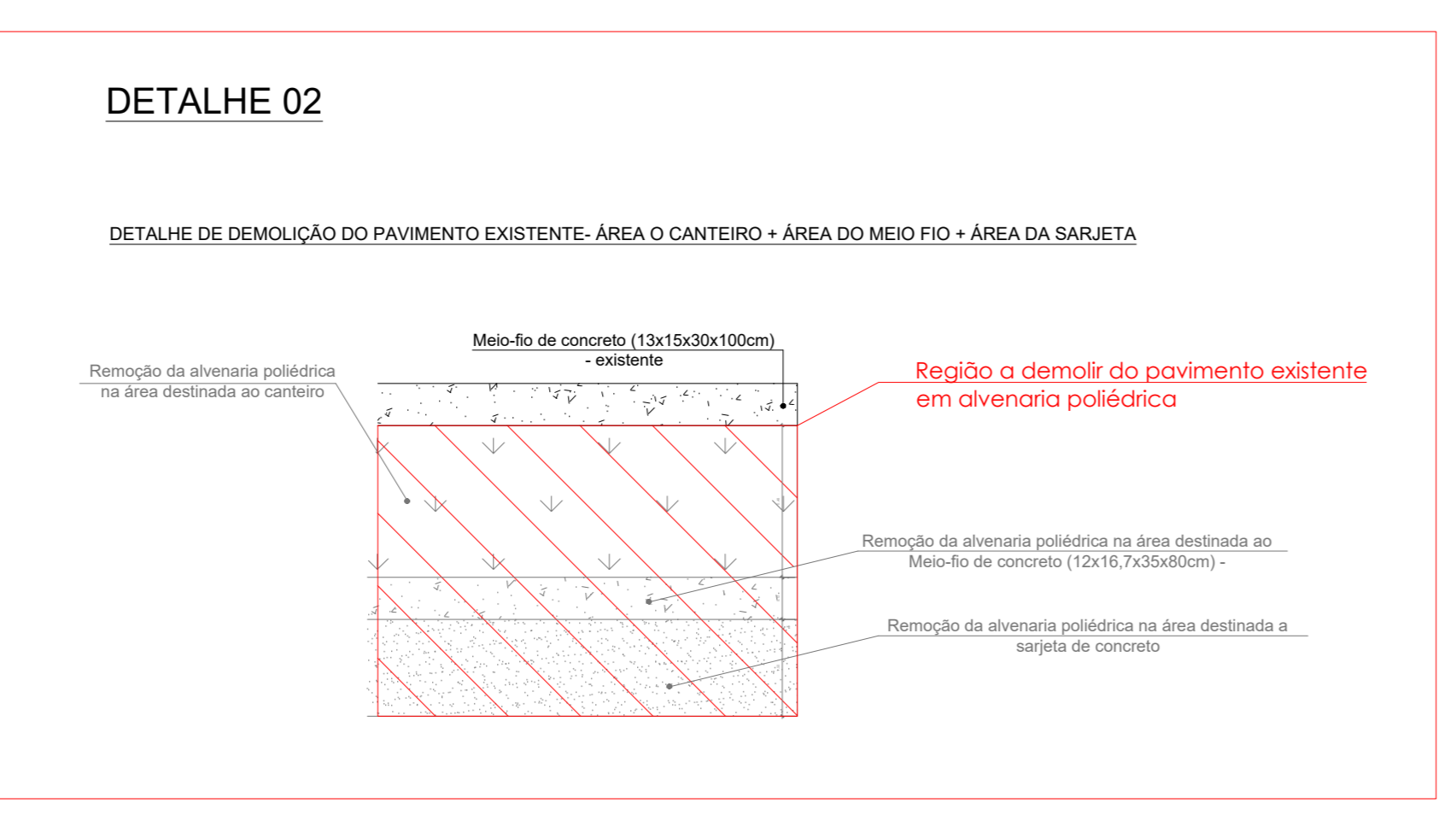
DETALHE DE DEMOLIÇÃO DO PAVIMENTO EXISTENTE
