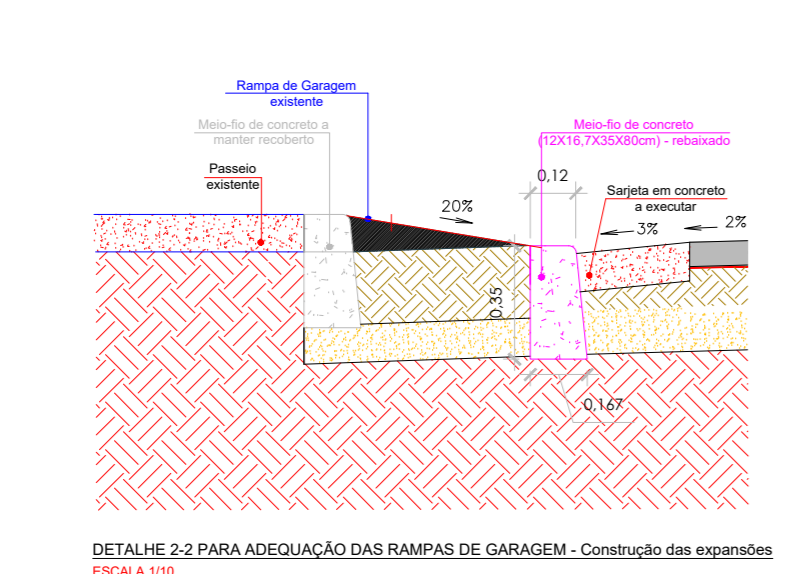
CORTE TRANSVERSAL DO DETALHAMENTO DA RAMPAS DE GARAGEM E CANTEIROS
