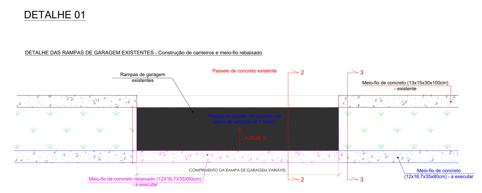
DETALHE DAS RAMPAS DE GARAGENS
