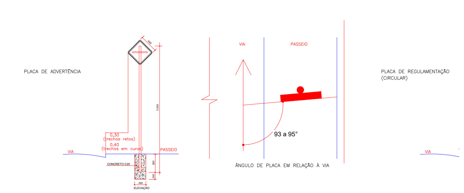
DETALHE SINALIZAÇÃO VERTICAL
